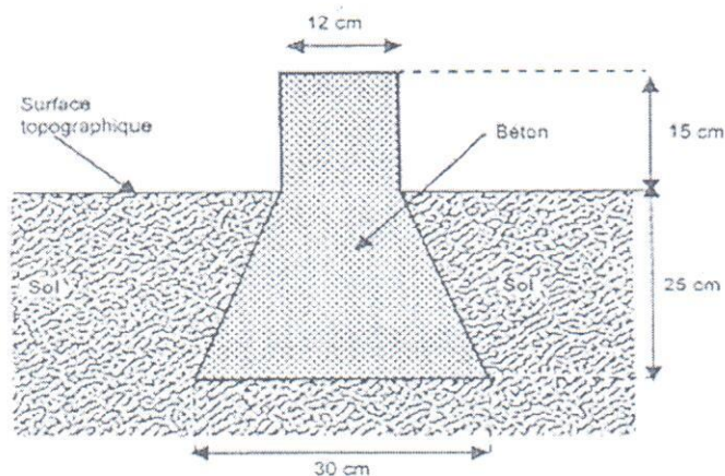
Point DFR/BL : coupe verticale de la borne
