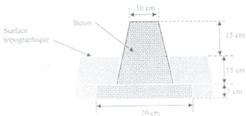
Point DFR/BT : coupe verticale de la borne
